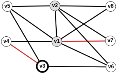
Слика 3.4: Пример случаја 1 када је d(v_r) - d_r = 1
