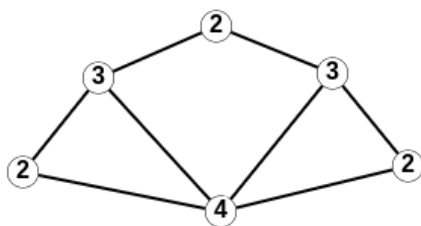
Слика 1.2: Граф који је реализација графичког низа \{4, 3, 3, 2, 2, 2\}
