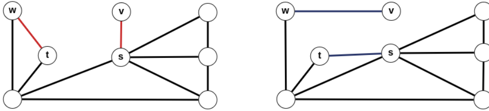
Слика 2.1: Замена грана код доказа теореме Хавела и Хакимија
