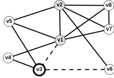
Слика 3.3: Пример случаја 1 када је d(v_r) - d_r = 2
