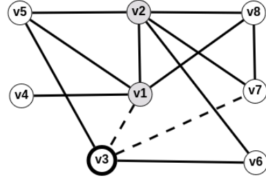
Слика 3.4: Пример случаја 1 када је d(v_r) - d_r = 1
