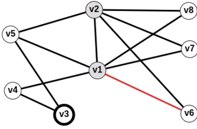
Слика 3.3: Пример случаја 1 када је d(v_r) - d_r = 2
