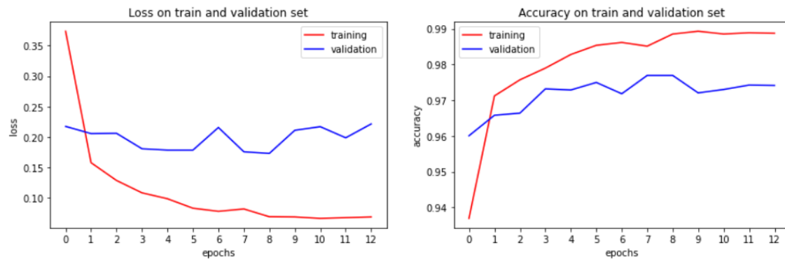
Slika 6.25: Obučavanje mreže - funkcija greške i tačnost
