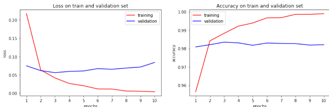
Slika 6.23: Obučavanje mreže - funkcija greške i tačnost
