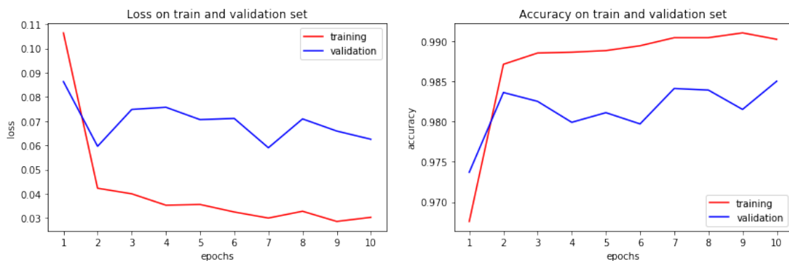
Slika 6.19: Obučavanje mreže - funkcija greške i tačnost
