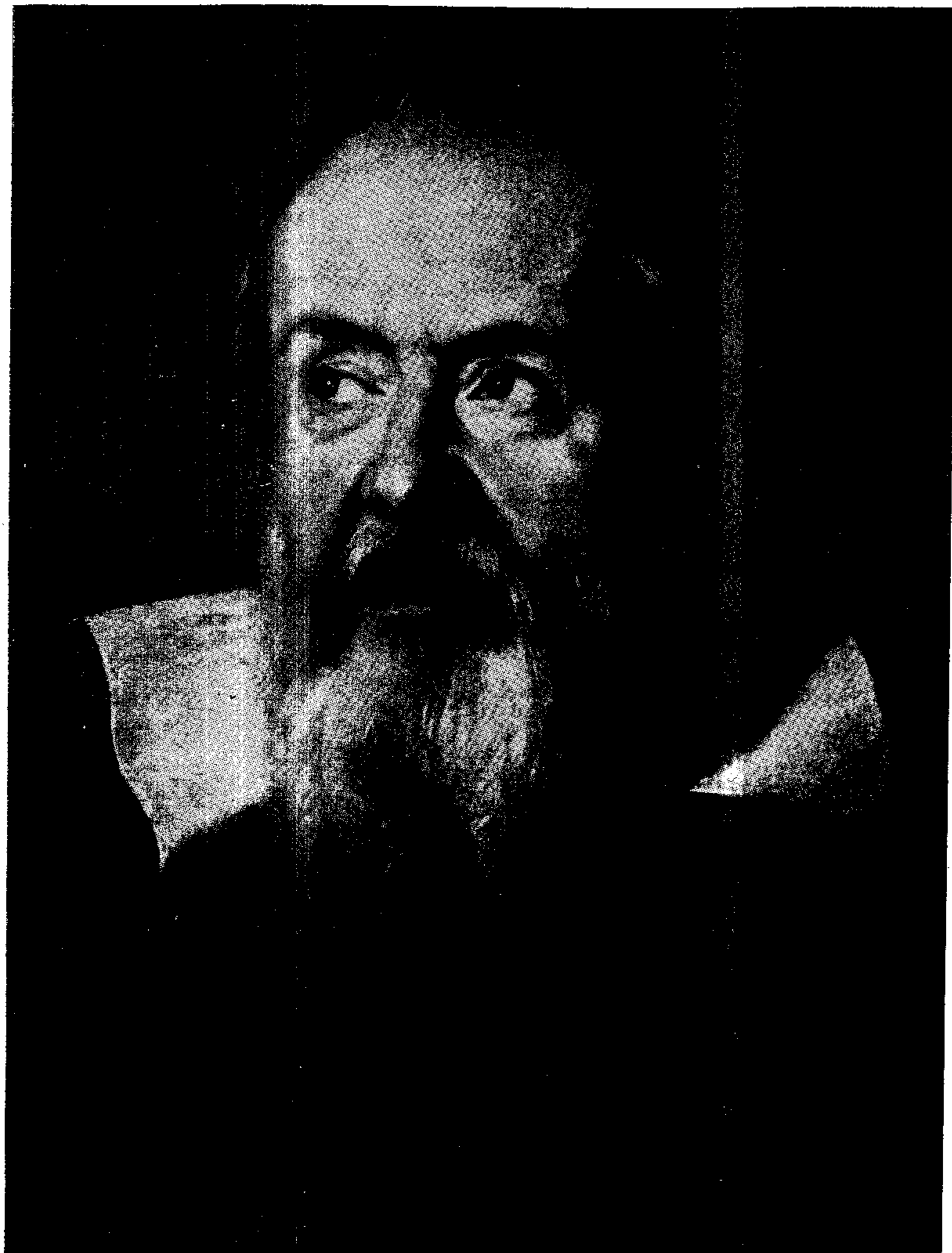
Галилео Галилеји 1564—1642
