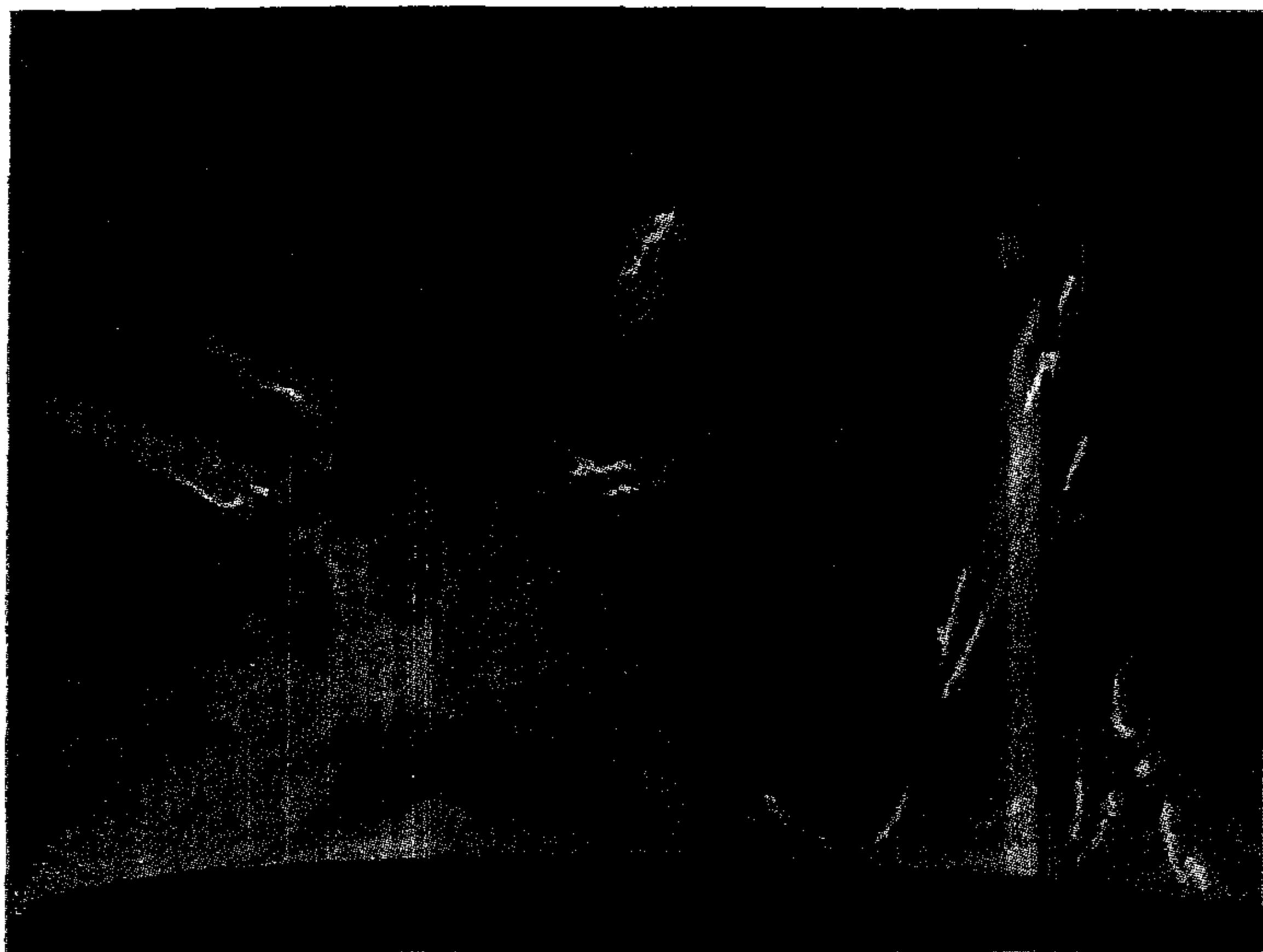
Сунчеве протуберанције
