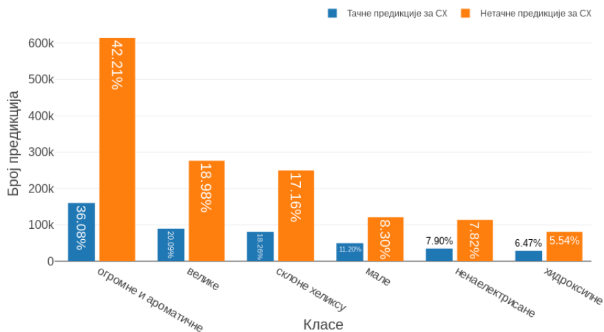
Слика 4.28: Однос тачних и нетачних предвиђања по класама за груписани биграма CX и num_of_max = 1
