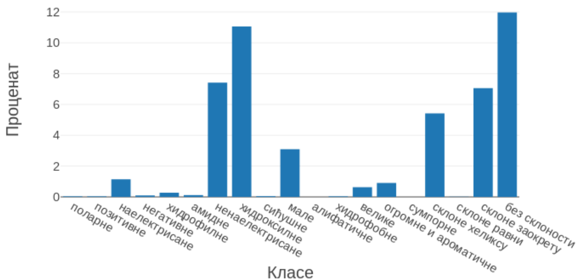
Слика 4.10: Проценат тачно предвиђених секвенци из тест скупа у односу на различите класе (праг је 65%)
