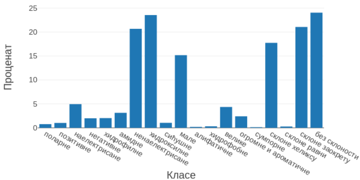
Слика 4.11: Проценат тачно предвиђених секвенци из тест скупа у односу на различите класе (праг је 50%)
