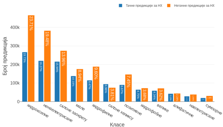
Слика 4.21: Однос тачних и нетачних предвиђања по класама за груписани биграма НХ и \text{num\_of\_max} = 1
