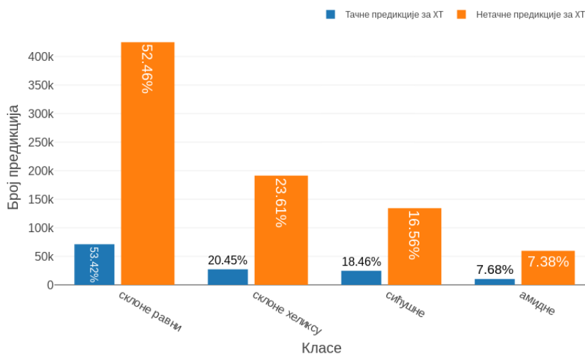
Слика 4.20: Однос тачних и нетачних предвиђања по класама за груписани биграма ХТ и \text{num\_of\_max} = 1
