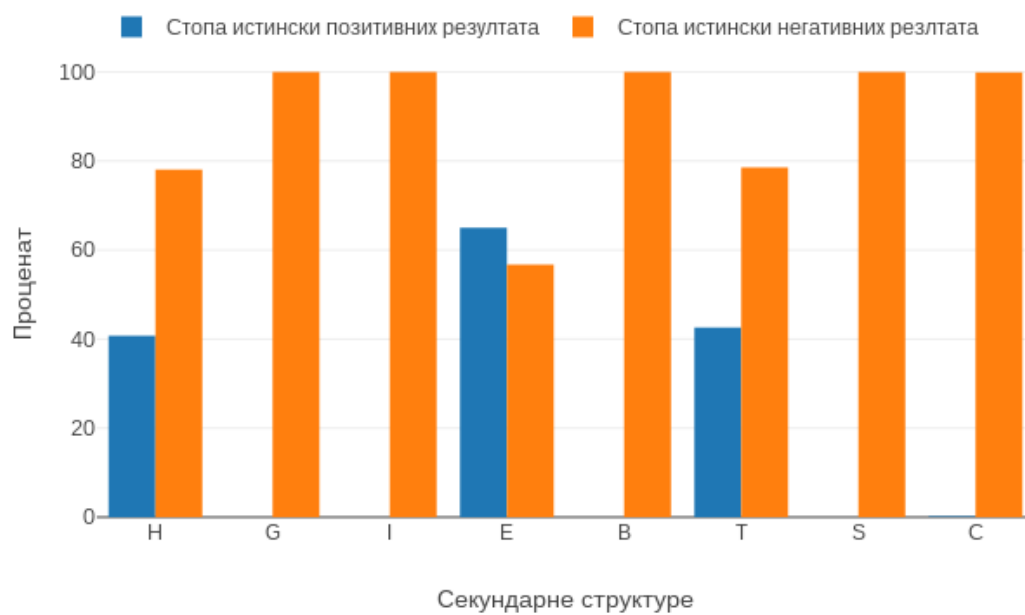
Слика 4.14: Однос вредности TPR и TNR за различите секундарне структуре и \text{num\_of\_max} = 3
