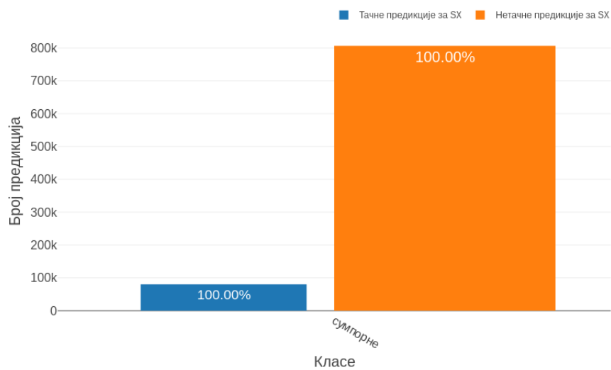
Слика 4.26: Однос тачних и нетачних предвиђања по класама за груписани биграм SX и num_of_max = 1
