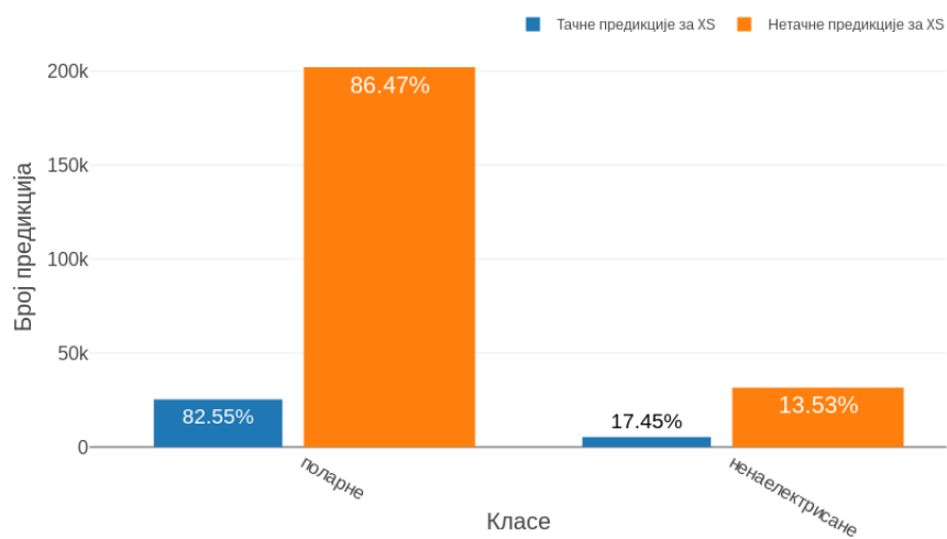
Слика 4.27: Однос тачних и нетачних предвиђања по класама за груписани биграм XS и num_of_max = 1
