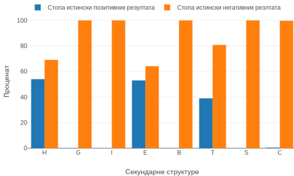
Слика 4.13: Однос вредности TPR и TNR за различите секундарне структуре и \text{num\_of\_max} = 2
