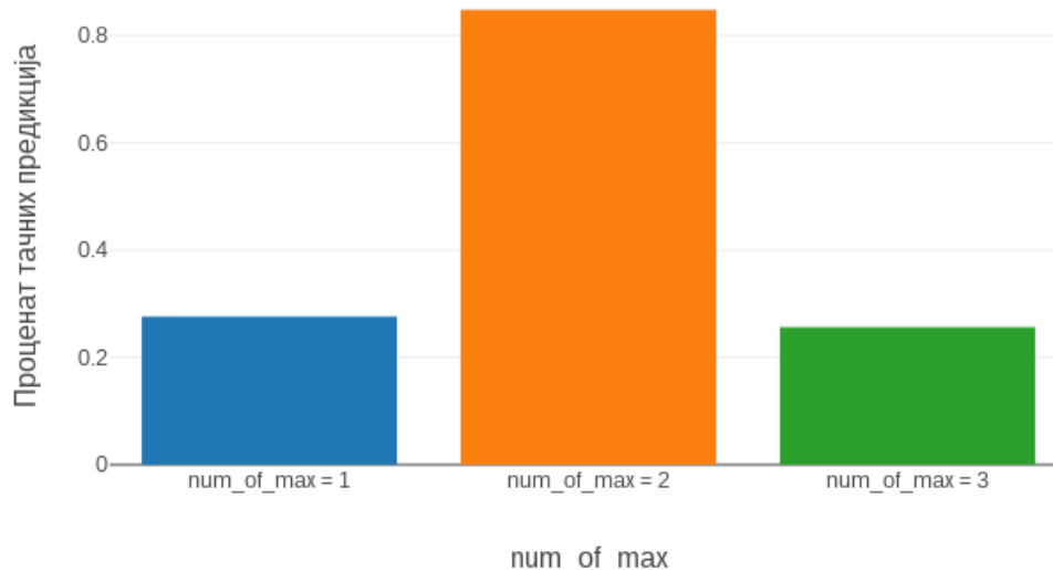
Слика 4.15: Проценат тачно предвиђених секвенци из тест скупа за различите вредности num_of_max (праг је 75%)
