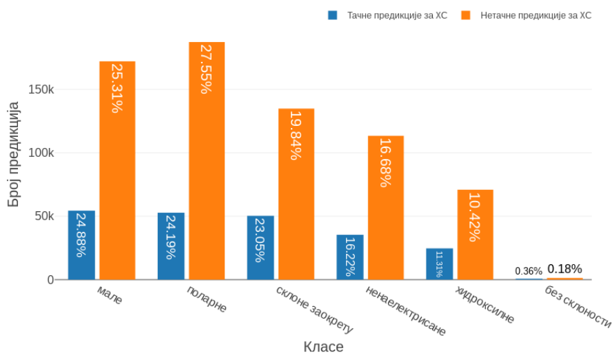
Слика 4.29: Однос тачних и нетачних предвиђања по класама за груписани биграма XC и num_of_max = 1
