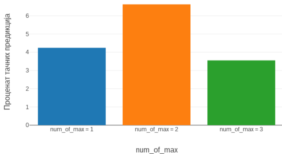
Слика 4.17: Проценат тачно предвиђених секвенци из тест скупа за различите вредности num_of_max (праг је 50%)
