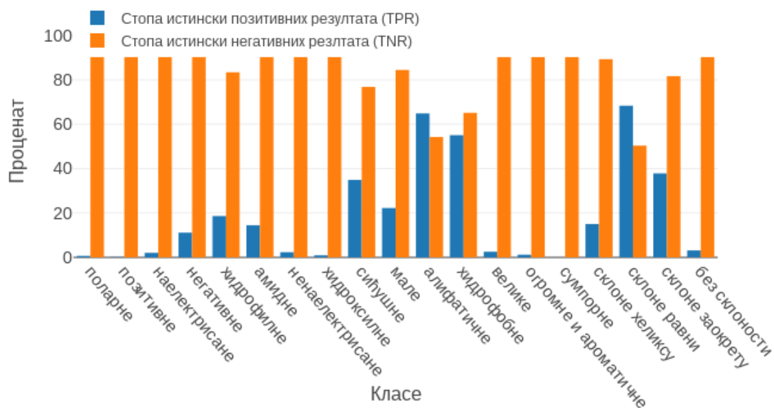
Слика 4.6: Однос вредности TPR и TNR за секундарну структуру T и различите класе
