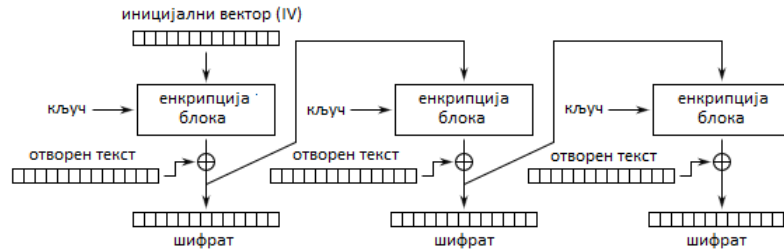
Слика 4: Шифровање подељених блокова коришћењем CFB
