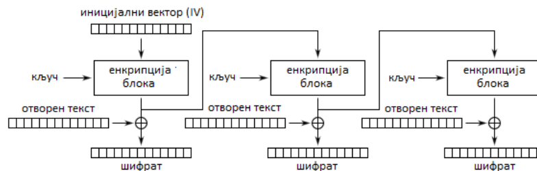
Слика 5: Шифровање подељених блокова коришћењем OFB
