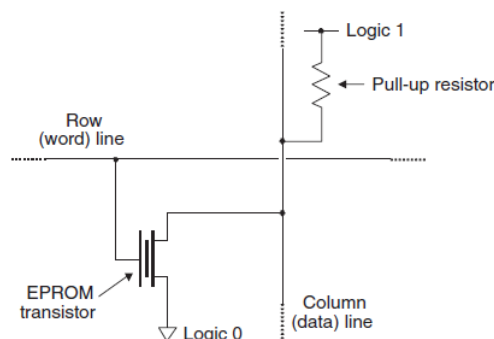
Слика 14: Пример EPROM ћелије FPGA чипа
