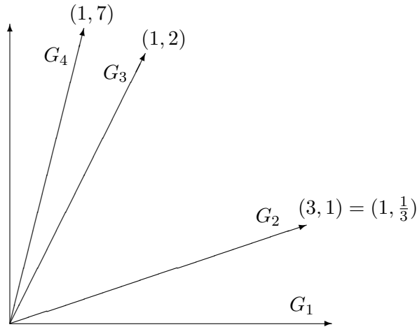
Figure 4.1: Gröbner fan for I
