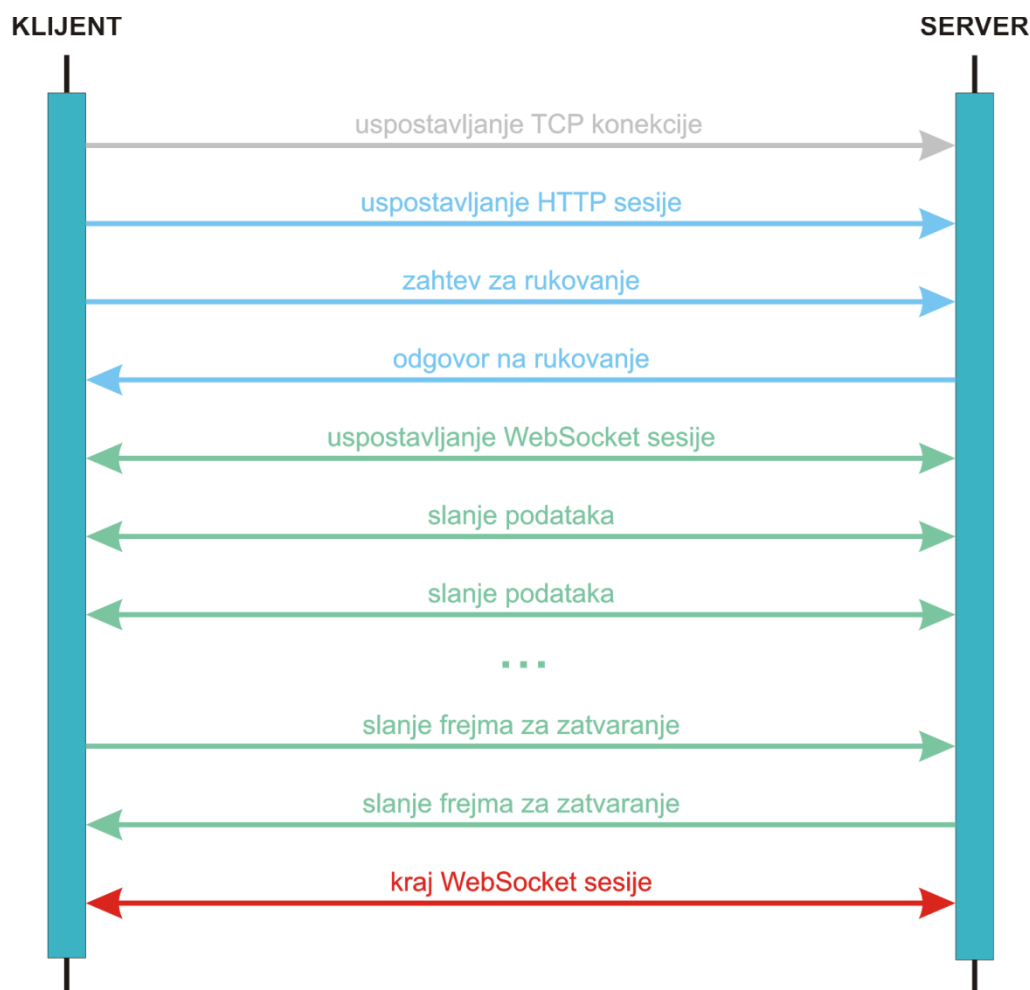
Slika 2-1 WebSocket protokol
