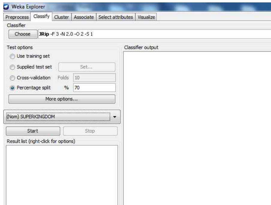
Слика 4.3: Радно окружење у WEKA-и након учитавња података који се класификују
