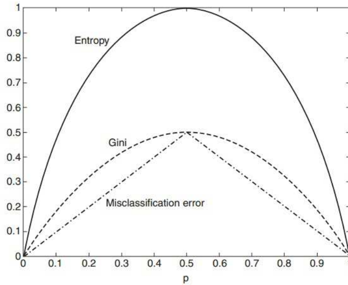
Слика 2.12: Упоредба мјера нечистоће
