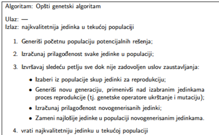
Слика 1 : Општи генетски алгоритам [5]
