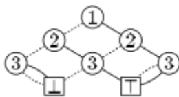
Слика 17: QDD Булове функције већинског одлучивања у примеру 24
