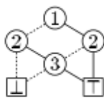
Слика 1: BDD репрезентација функције већинског одлучивања са три променљиве из примера 1
