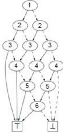
Слика 16: Функција већинског одлучивања T_3^6 из примера 21
