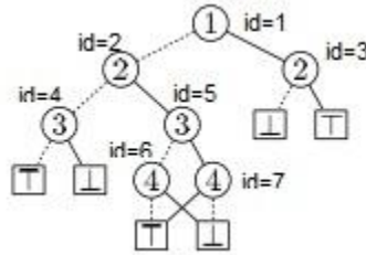
Слика 11: BDD из примера 16
