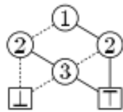
(а) Редукован уређен BDD
