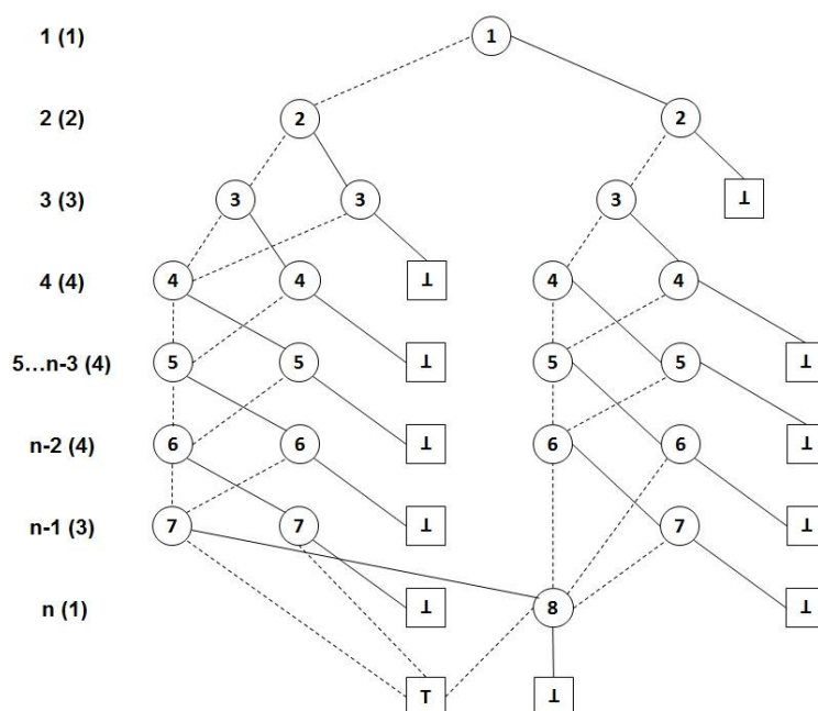
Слика 13: BDD независних скупова циклуса C_8
