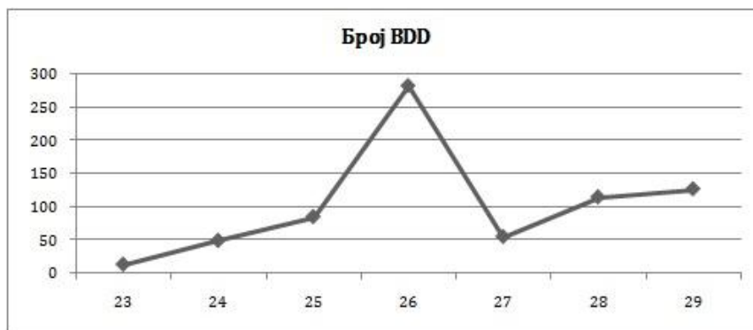
Слика 20: Расподела броја чворова и броја BDD истинитосне табеле (103)
