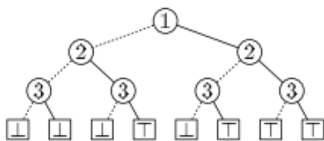
(а) Нередукован граф
