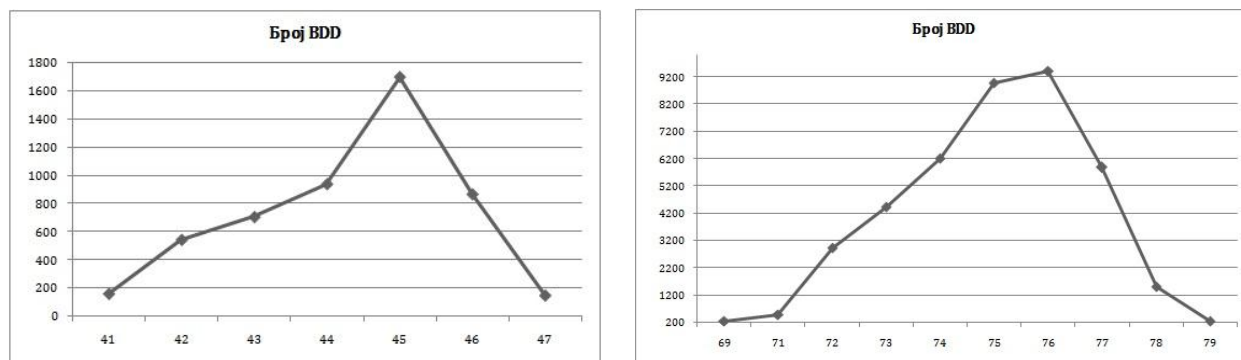
Слика 21: Расподела броја чворова и броја BDD за n = 7 и n = 8 . За истинитосне табеле из (104) важи да:
