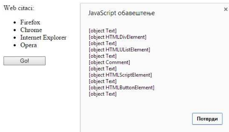
Слика 24. Потомци елемента <body>
