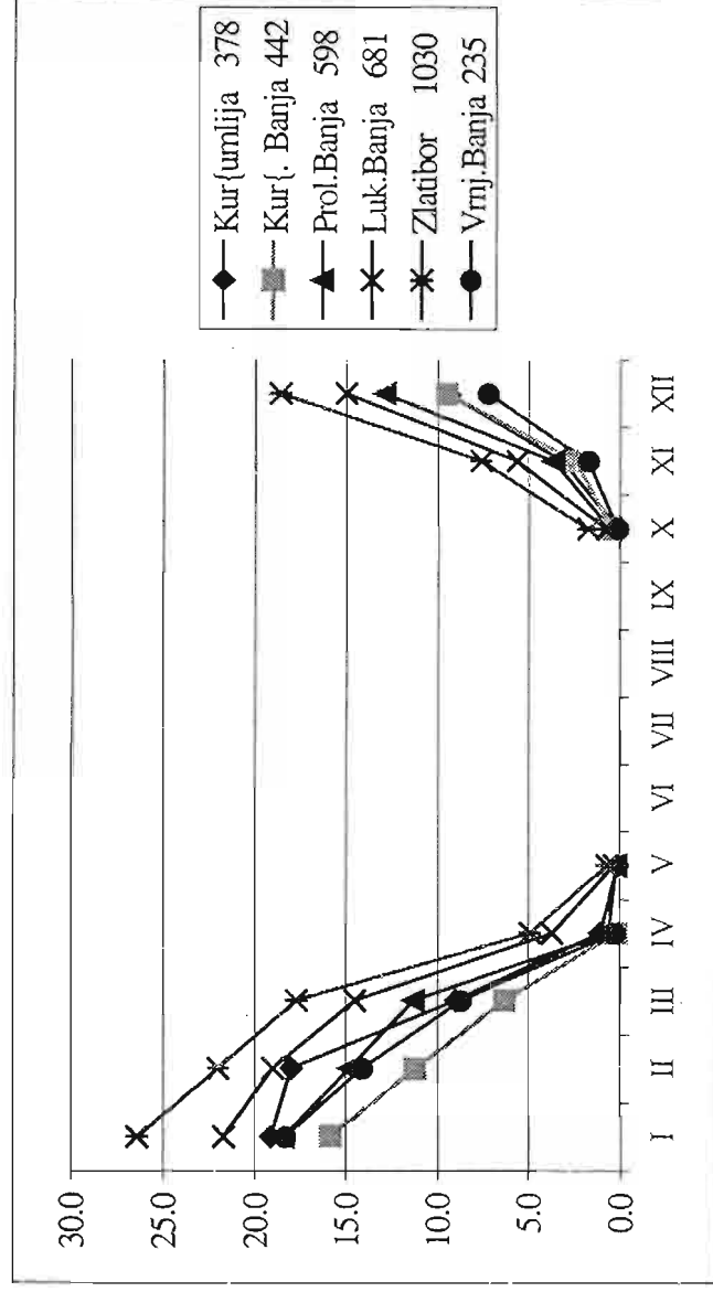
Графикон 6. Годишњи ток снежног покривача
