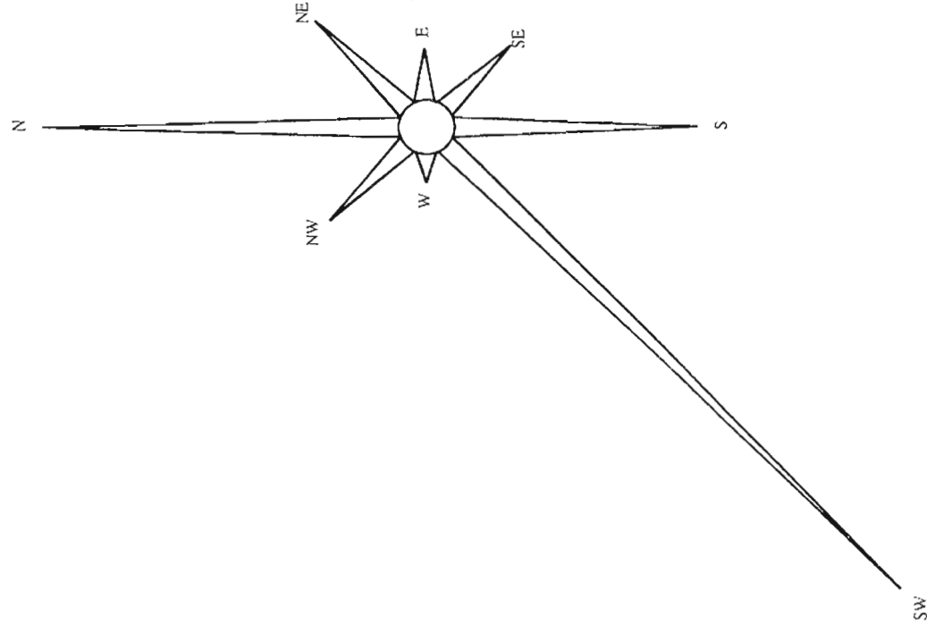
Графикон 4. Ружа ветрова за Куршумлију (период 1961-1990.год.)
