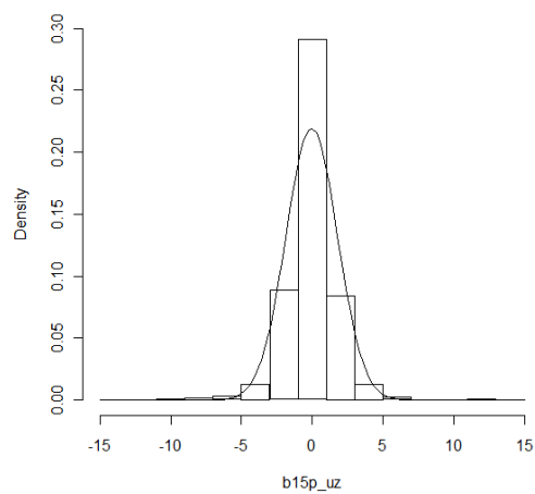
Normalna raspodela i histogram prinosa iz uzorka
